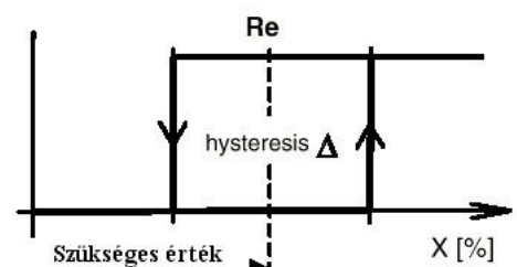
DIR 140 A karakterisztikája
