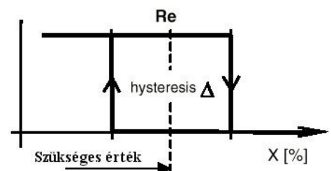
DIR 140 B karakterisztikája
